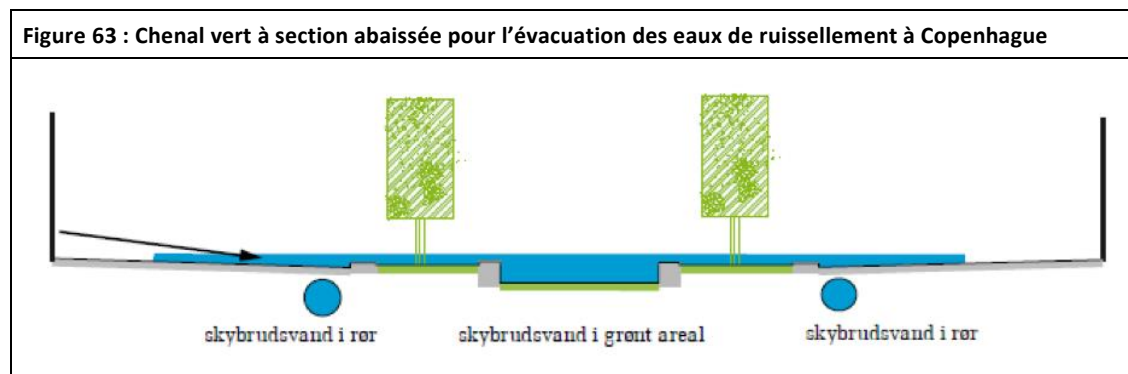
Exemple de chenal vert à section abaissée pour l'évacuation des eaux de ruissellement (source : Nielsen 2013)
